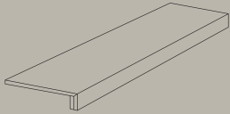
SCALINO INCOLLATO GLUED STEP TREAD / NEZ DE MARCHE COLLÉ / GEKLEBTE STUFENPLATTE / PELDAÑO CON PERFIL PEGADO ▲ 30x120 (13"x48") RT 20mm
